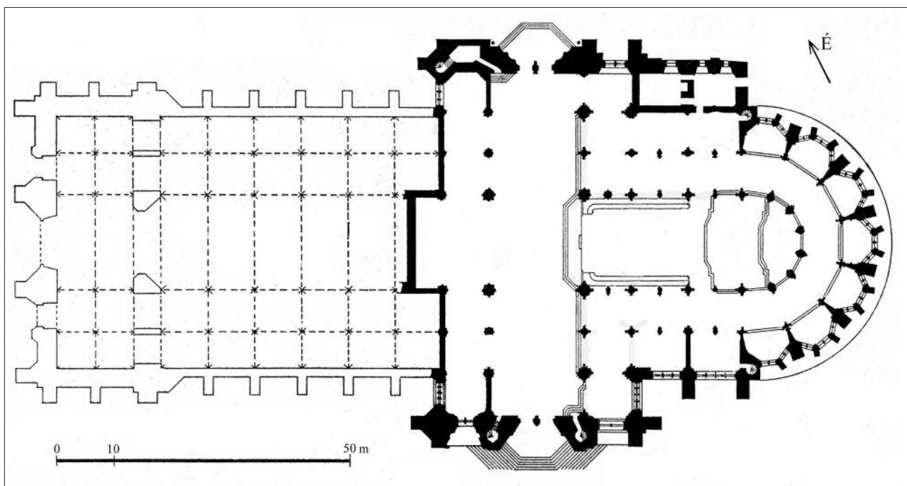
1. ábra. A székesegyház alaprajza
