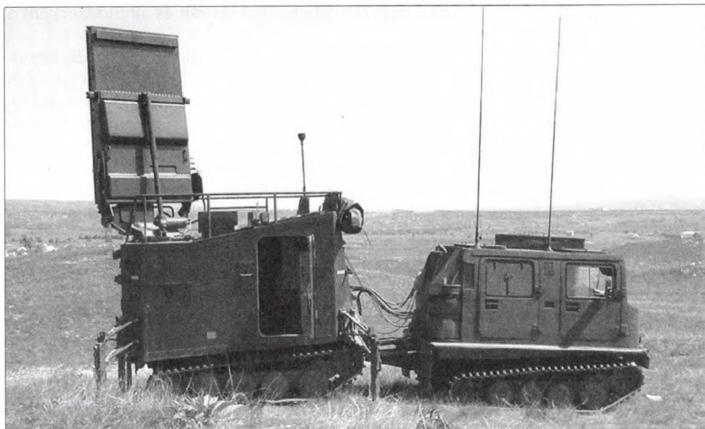
1. kép. ARTHUR Tüzérségi Felderítő Radarrendszer – BV 206 vontatott változat
