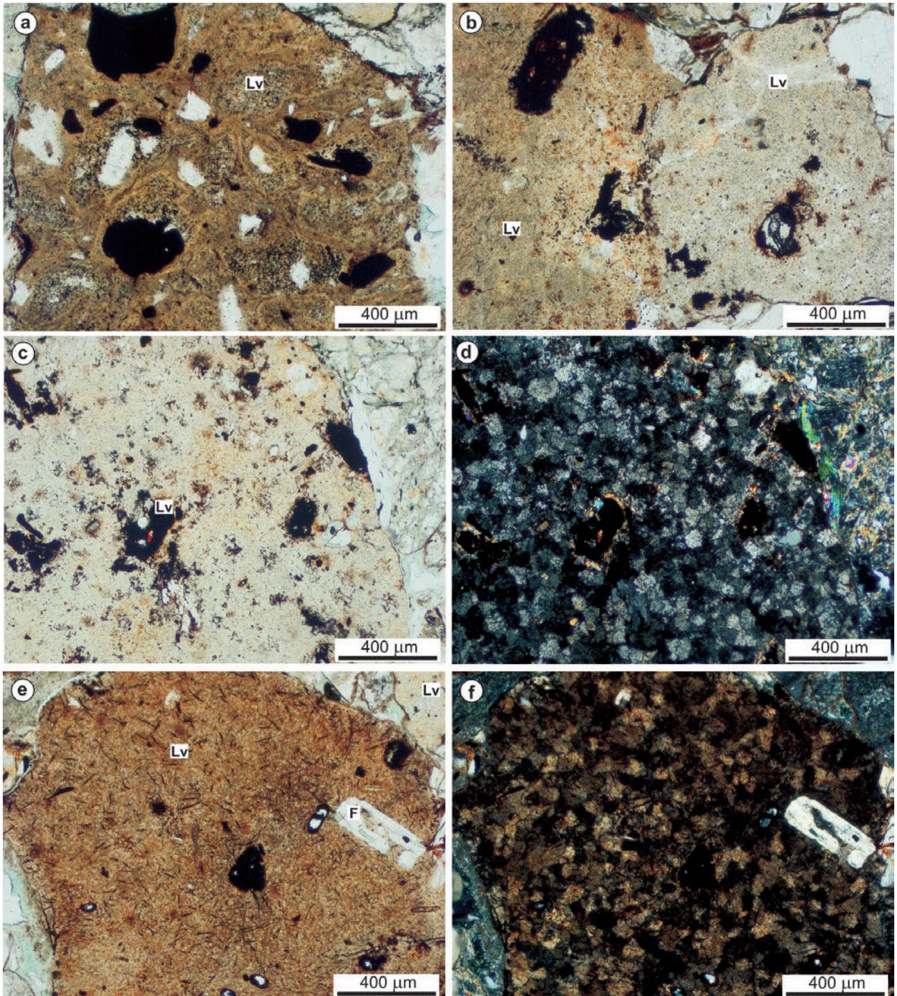
10. ábra. A 9. vékonycsiszolat petrográfiai jellemzői (a–c és e: 1N; d és f: +N), 9012. sz. fúrás, Cserdi Formáció. a) Átkristályosodott, reliktvitroklasztos szövetű vulkáni kőzettörmelék; b–f) Különböző megjelenésű, felzitesen átkristályosodott vulkanitszemcse
