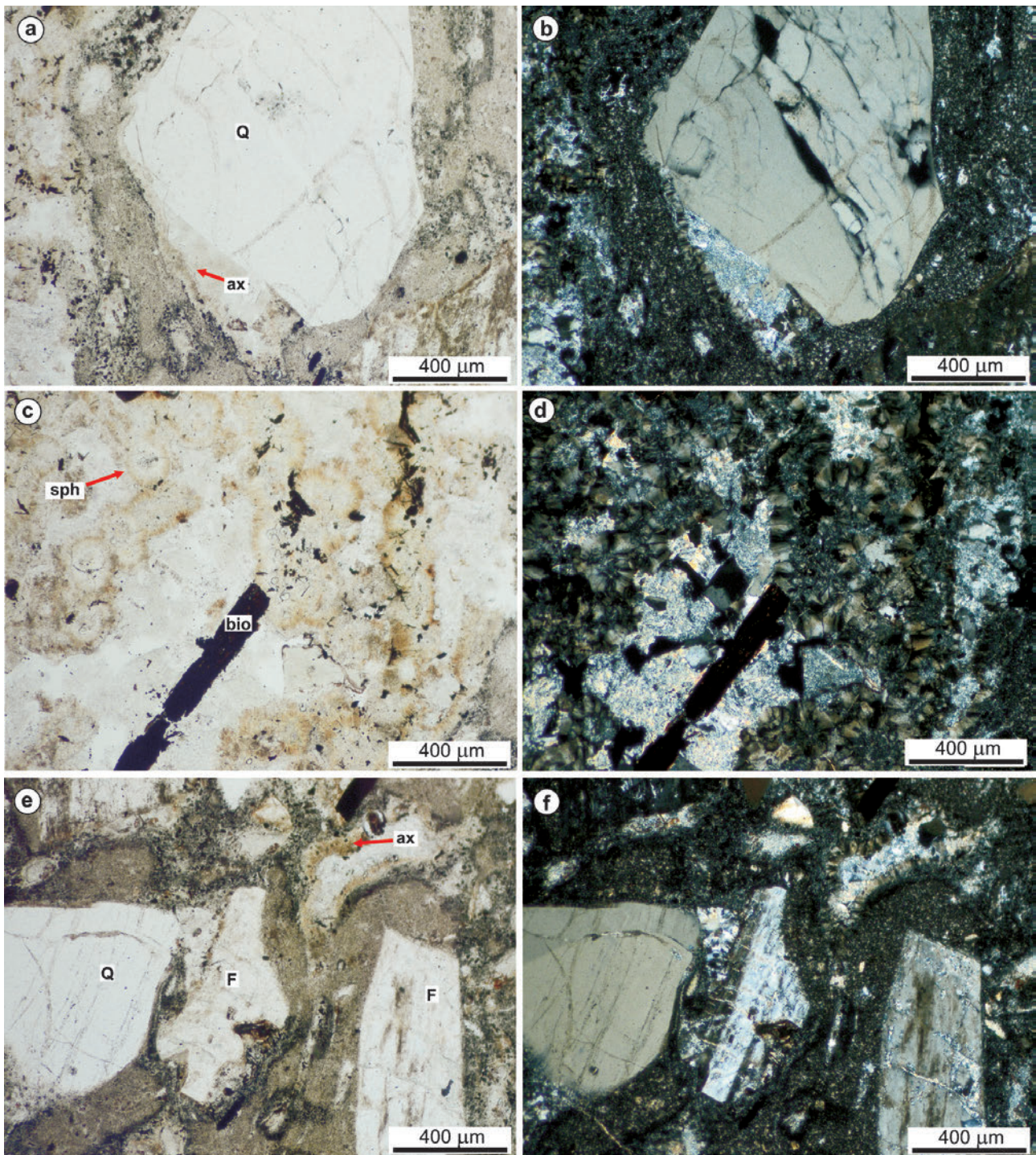
6. ábra. A 3. vékonycsiszolat petrográfiai jellemzői (9007. sz. fúrás 119,5 m, Gyűrűfüi Riolit Formáció). a) és b) Törött és sűrűn repedezett kvarc fenokristály, a repedések mentén fluidumzárványosorokkal. Szegélyére egykori üveges olvadék tapadt (nyíl), mely devitrifikálódott, széle axiolitosodott (1N és +N); c) és d) Az egykori üveges horzsakő belső üreges mikroszerkezete teljesen átalakult, belsejében gömb (nyíl) és legyező alakú szferulitok figyelhetők meg (1N és +N); e) és f) Az erősen átkristályosodott alpanyag törött kvarc és földpát fenokristályokat, biotitot, illetve átalakult horzsakőszilánkokat tartalmaz. Az egykori horzsakőszilánkok barna szegélyét axiolitos devitrifikáció eredményeként kristályosodott földpát alkotja, belsejüket finomkristályos kvaremozaik tölti ki (1N és +N) Rövidítések: Q: kvarc; F: földpát; bio: biotit, illetve biotit utáni opak pszeuomorfóza; ax: axiolitos devitrifikáció; sph: gömbös szferulit
