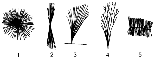
3. ábra. A szferolitok morfológiai típusai MCPHIE et al. (1993) alapján módosítva
