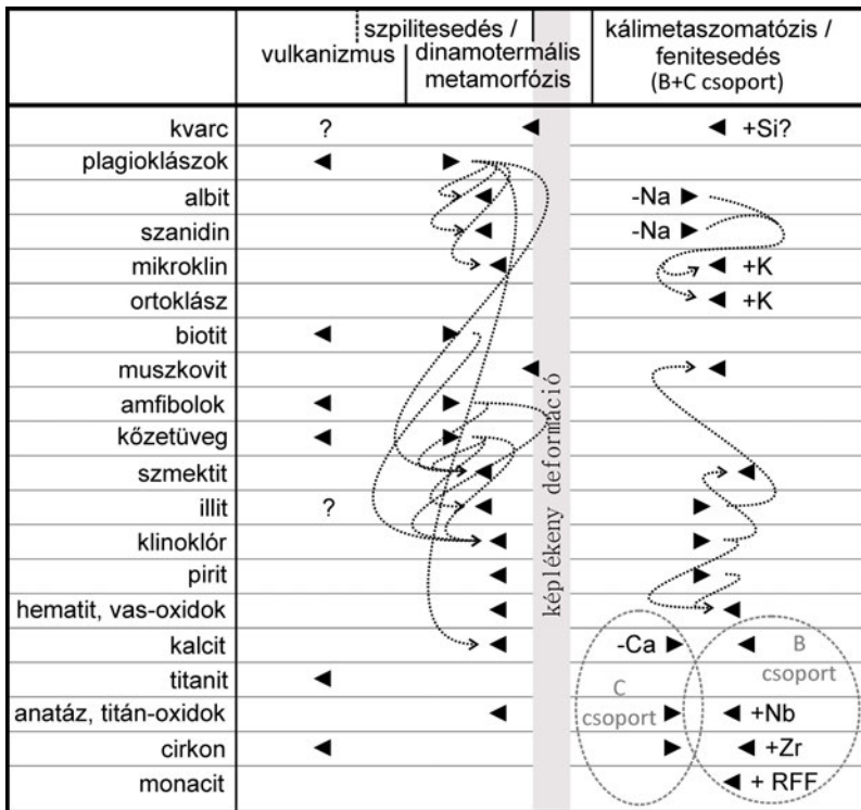
7. ábra. A jellemző ásványok, szövetalkotók képződésének és átalakulásának genetikai összefüggései. ◀ – ásványképződés, ▶ – átalakulás és helyettesítés a nyílal összekötött képződő fázisokkal, ? – bizonytalan, de a kőzetek egy részében feltehető képződés, ±M – fém hozzáadódása külső forrásból, vagy fém távozása
