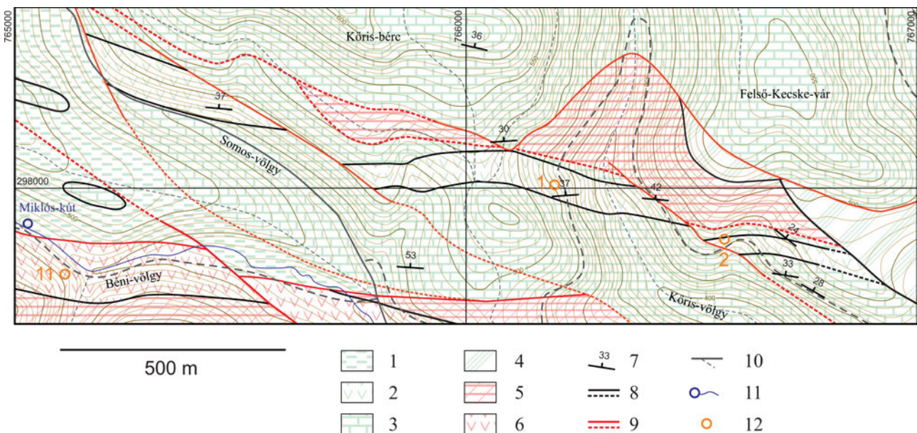
2. ábra. Földtani térkép a Kőrös-völgyi ritkaelem-dúsulást hordozó metavulkanit-kibúvásról Zöld sraffozás - Bükk-szentkereszt-tektofácieshez tartozó kőzettestek: 1 – aleurolitpala (Lök-völgyi F), 2 – metavulkanit (B csoport) (Szinvai Metabazalt F), 3 – tűzköves mészkő (Felsőtárkányi Mészkő F), 4 – tűzkőtörmelék (málladékkal fedett terület). Rózsaszín sraffozás - Kácsi tektofácieshez tartozó kőzettestek: 5 – cukorszövetű dolomit (Belvácsi Dolomit T), 6 – metavulkanit (C csoport) (Szentistvánhegyi Metaandezit F). Egyéb jelek: 7 – palásság, 8 – rátelepüléssel, 9 – tektonikus kontaktus, térképezett és valószínűsített, 10 – utak, 11 – forrás és patak, 12 – elemzett minták származási helyei
