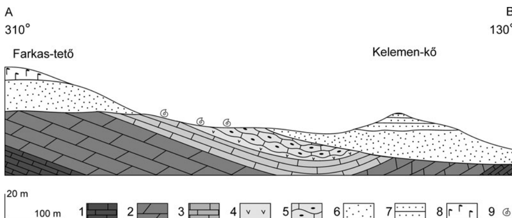
3. ábra. A szentbékkállai kőtegyer (Kelemen-kő) és a Farkas-tető közötti terület földtani szelvénye (A-B nyomvonala a 2. ábrán) 1 – Iszkahegyi Mészkő Formáció (alsó-anisusi), 2 – Megyehegyi Formáció (alsó-anisusi), 3 – Felsőörsi Mészkő Formáció (középső-felső-anisusi), 4 – Vászolyi Formáció (felső-anisusi), 5 – Buchensteini Formáció (ladin), 6 – Kállai Formáció, homok (felső-miocén), 7 – Kállai Formáció, kovás homokkő (felső-miocén), 8 – Tapolcai Bazalt Formáció (felső-miocén-pliocén), 9 – ammonitesz-lelőhely
