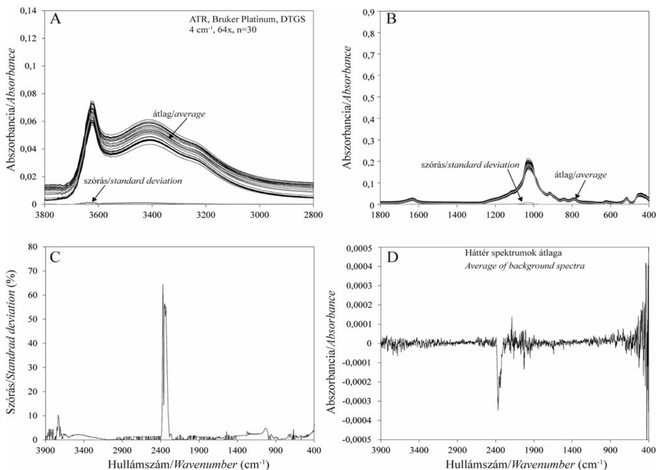
5. ábra. Az STx-1b agyagásvány-sztenderd 30 különböző mintaadagjának spektrumai a 2800–3800 \text{cm}^{-1} (A) és a 400–1800 \text{cm}^{-1} (B) közötti hullámszámtartományban. Az ábrán feltüntetjük az átlag és szórás spektrumokat is szürke vastag vonallal. A felvételek Bruker Vertex 70 spektrométerrel, Bruker Platinum ATR egységgel és DTGS detektorral készültek. A spektrumokon bővített ATR korrekciót alkalmaztunk. A C ábrán az egyes hullámszámoknál tapasztalható szórás%-ot mutatjuk be. A D ábra 30 üres mintával felvett mérés átlag spektrumát mutatja be.
