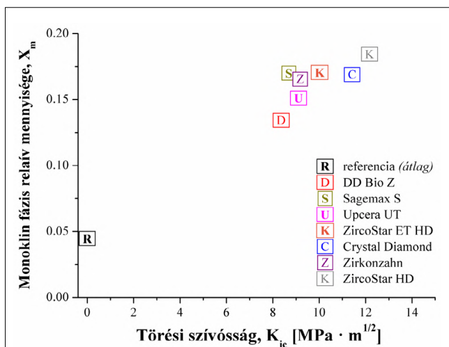
6. ábra: A törési szívóssághoz tartozó, az egyes mintatípusok törési felületein meghatározott monoklin fázis mennyiségeket ábrázoltuk.
