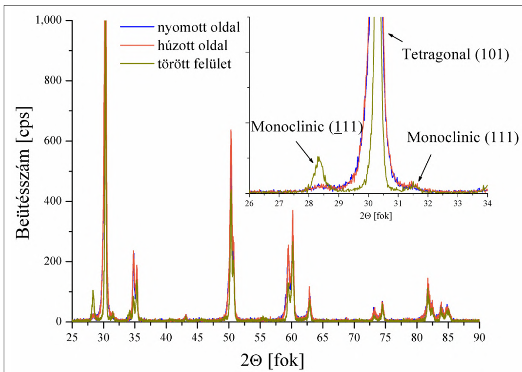
4. ábra: Y-ZrO kerámia monoklin – tetraclin fázis görbéje a hajlítószilárdsági próbatest húzott, illetve nyomott felületeiről
